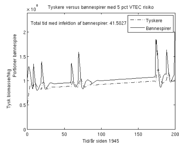
Figur 1: Middelværdier med standardafvigelse for antallet forureningsperioder over 200 år ved forureningsrisiko på 1-5 pct. Figurene viser plots over tidsudviklingen af bønnespire- og tyskerbiomasse ved p = 1, 4, 5 pct forureningsrisiko.
